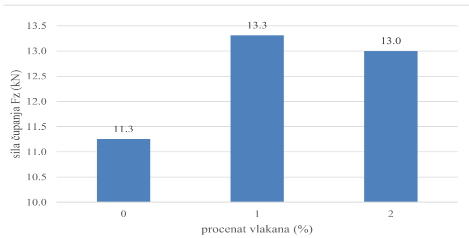
Slika 7 – Rezultati ispitivanja putem pull-off testa (0, 1 i 2% vlakana, CEM I 52,5R)
